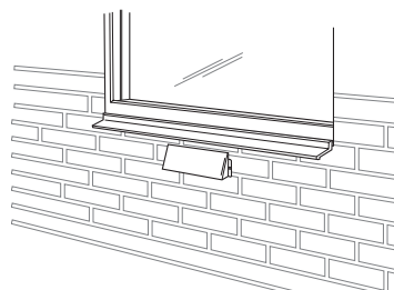
5. Montering av fasadgaller
