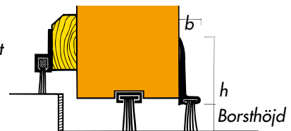
Sektion innerdörr/entréport
